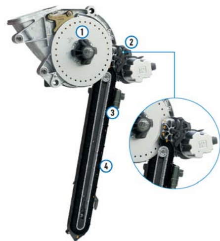
Zaujímavá a jedinečná ASG doprava osiva kefovým dopravníkom. Jeho rýchlosť sa prispôbuje pojazdovej rýchlosti.
